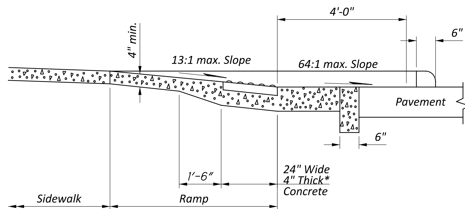
SECTION D-D
