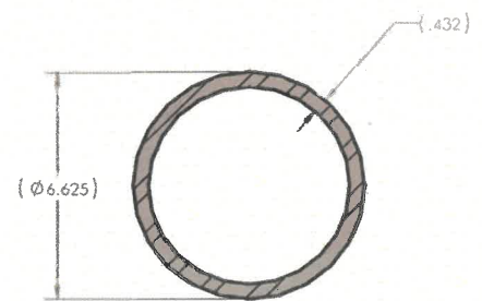
SECTION A-A SCALE 1 : 3
